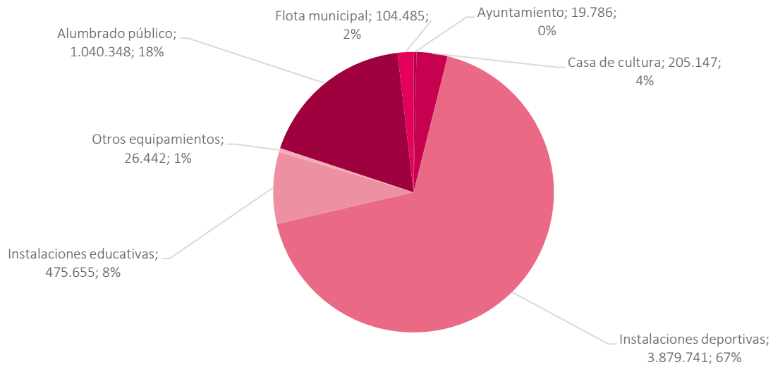
Figura 10 Consumo municipal total de energía final por uso (kWh) Huarte/Uharte, 2023 7 .
