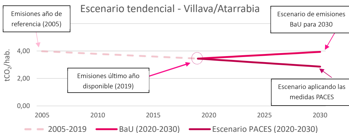
Figura 23 Gráfico de escenarios tendenciales para Villava/Atarrabia
