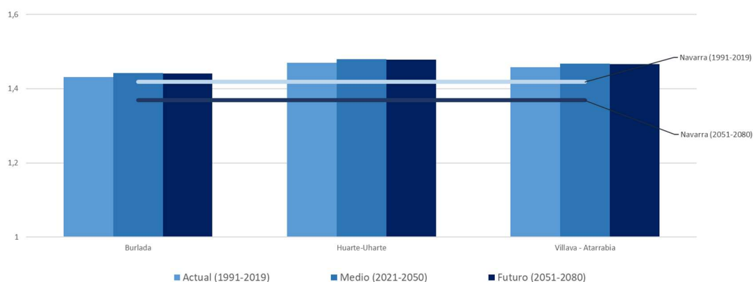
Figura 26 Evolución del riesgo frente a inundaciones
