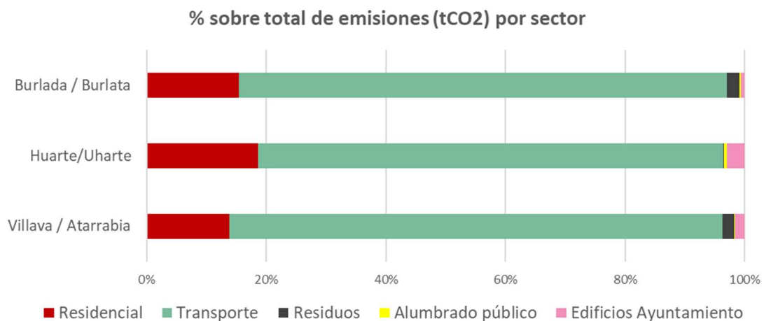
Figura 17 Distribución de emisiones (tCO 2 ) por sector sobre total del municipio, 2019
