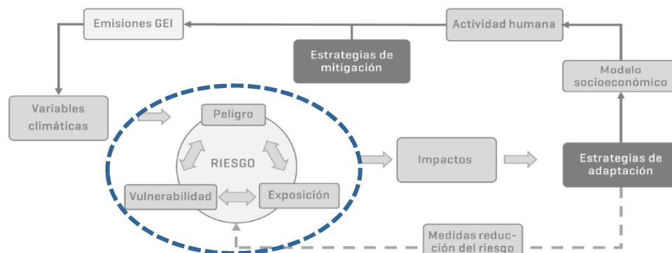
Figura 25 Metodología del análisis de vulnerabilidad y riesgo frente al cambio climático
