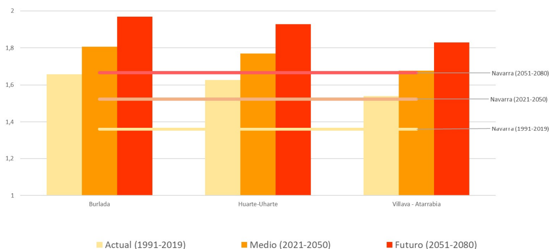
Figura 27 Evolución del riesgo frente a temperaturas extremas
