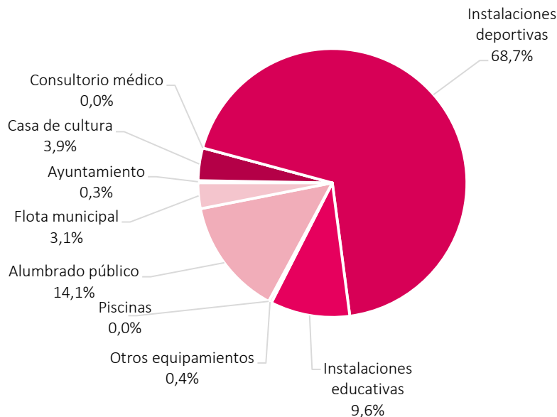
Figura 21 Emisiones municipales (kgCO 2 ) Huarte/Uharte, % por uso
