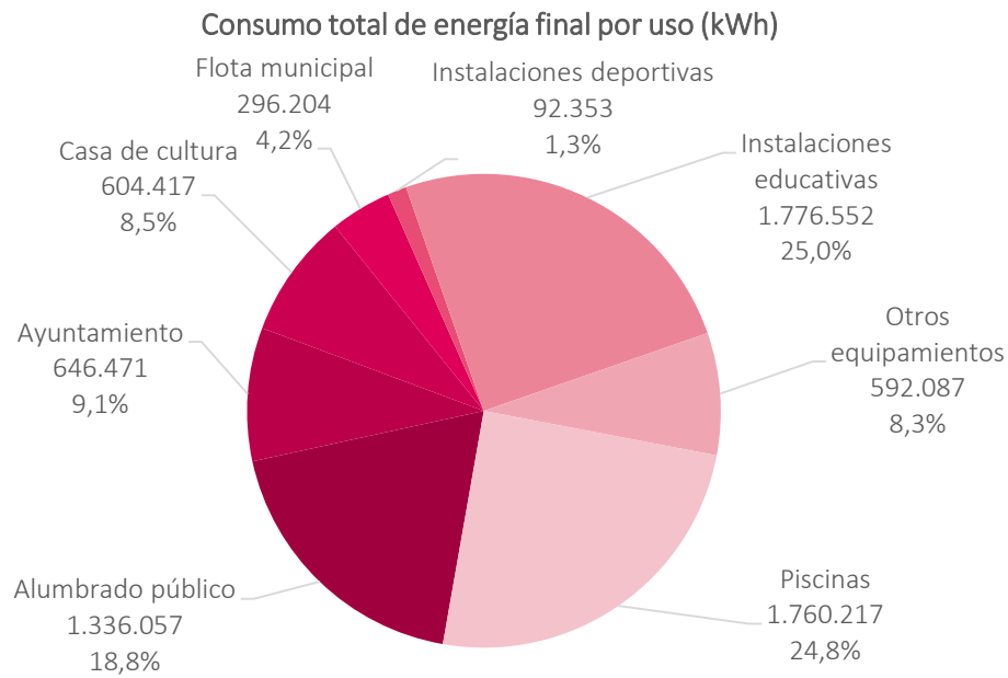
Figura 9 Consumos energéticos del sector municipal de agrupación, por uso 6 .
