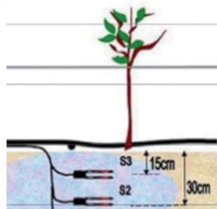
Figura 3. Sondas de control de Humedad suelo
