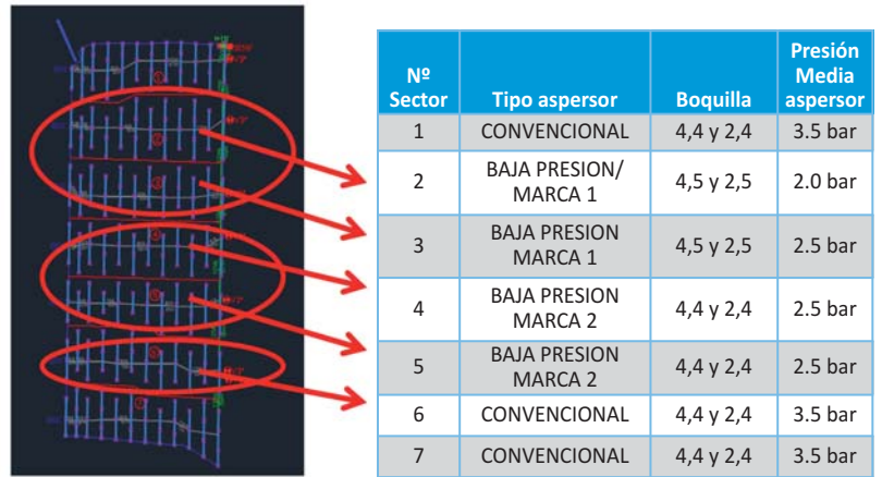
Figura 2. Ensayos de aspersores a baja presión
