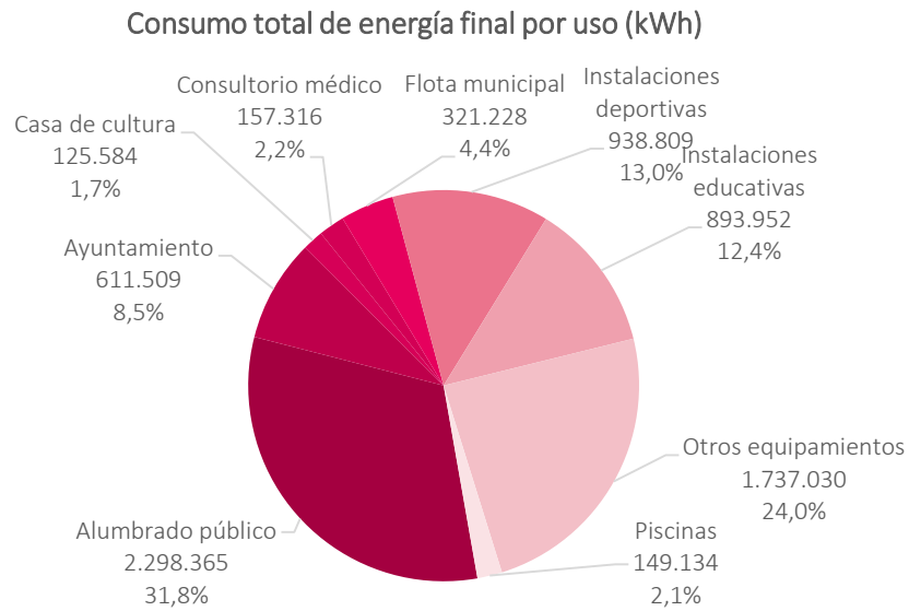
Figura 10 Consumos energéticos del sector municipal de la agrupación, por uso 10
