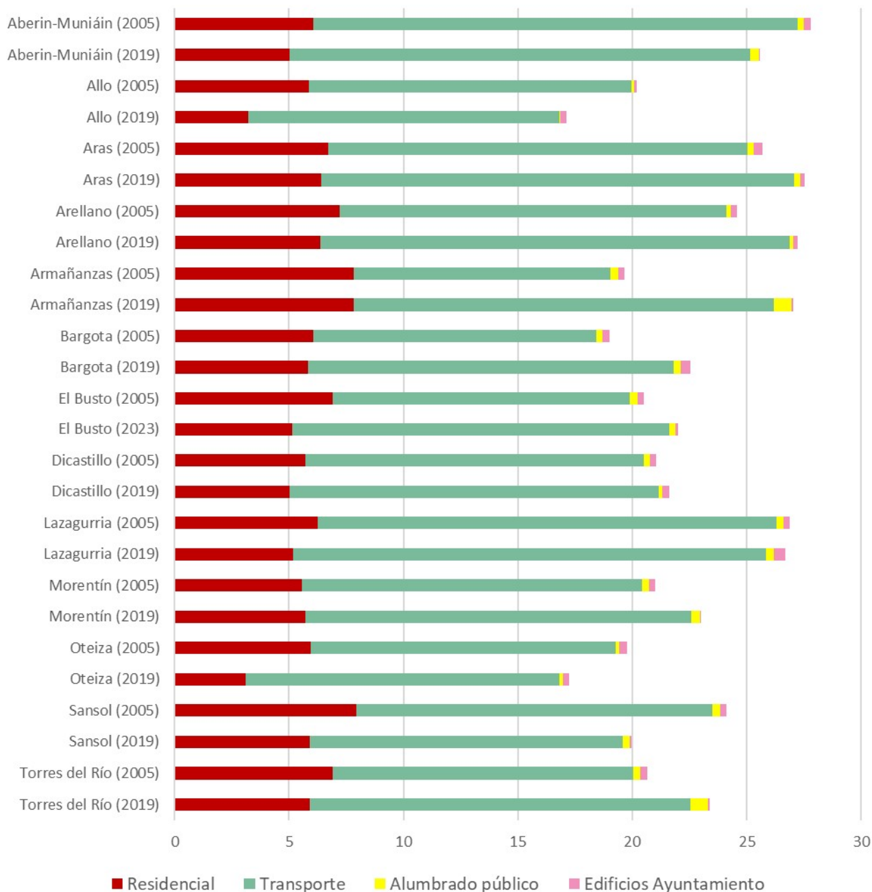
Figura 7 Evolución de los consumos por habitante (MWh/hab) para municipios <1.000 habitantes.
