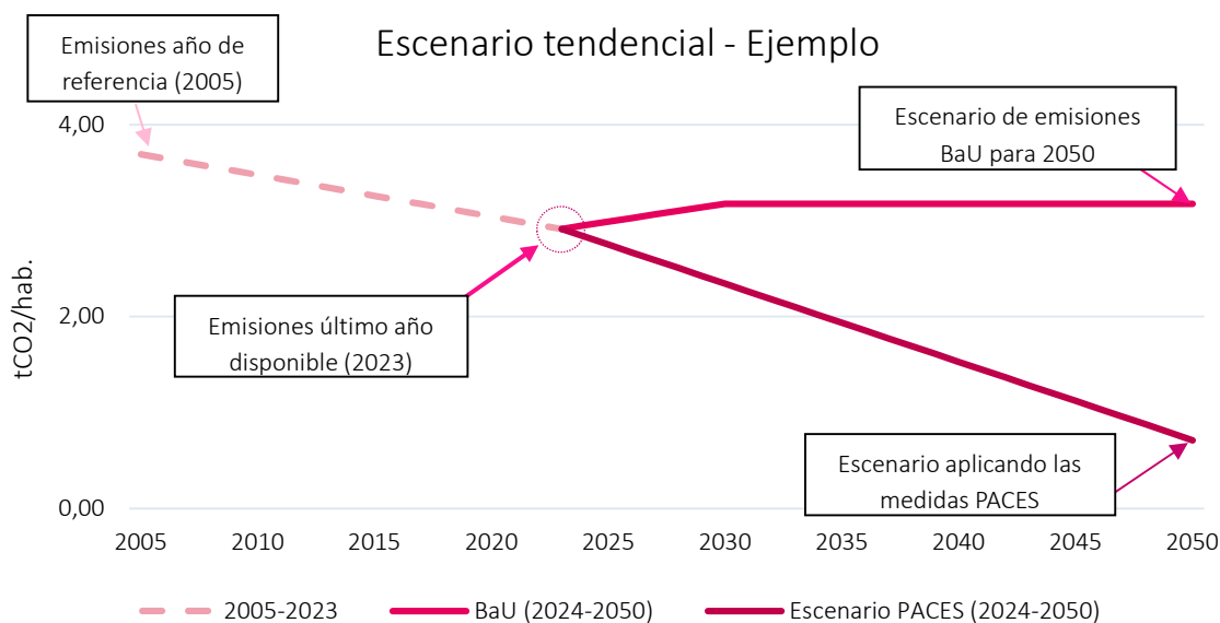
Figura 25 Ejemplo de gráfico de escenarios tendenciales 2050 del Anexo VI
