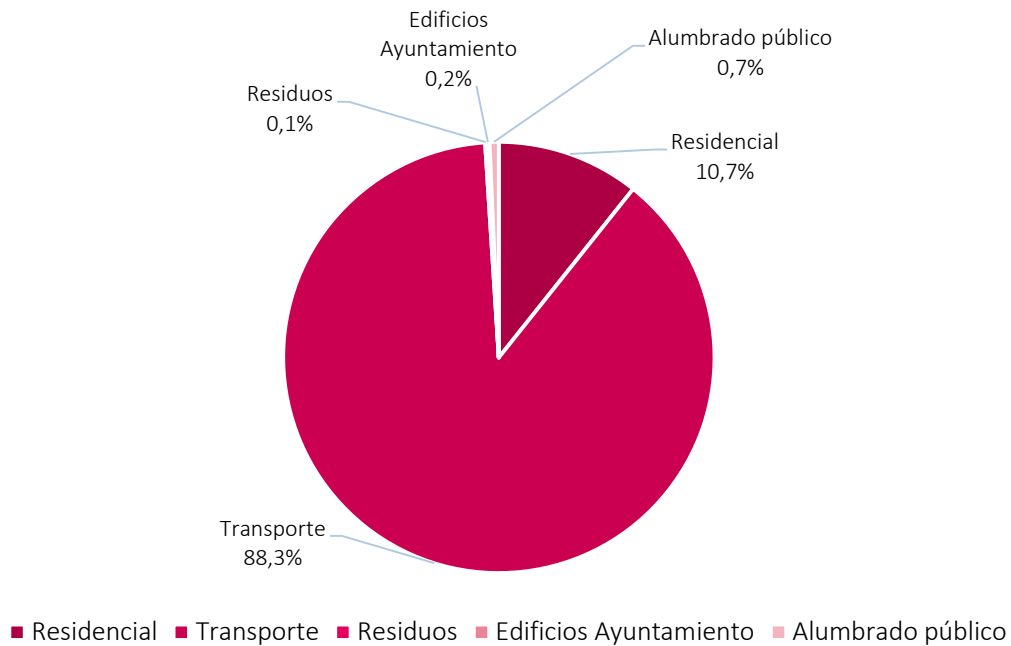
Figura 21 Emisiones (tCO 2 ) de El Busto, por sector
