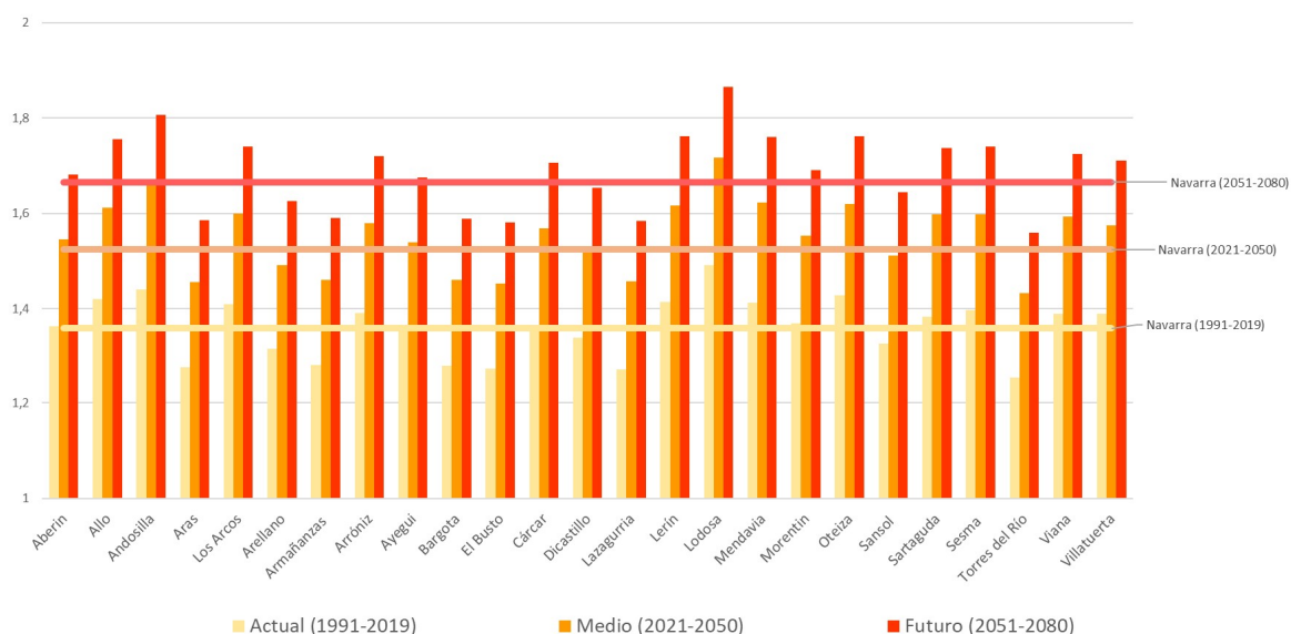
Figura 28 Evolución del riesgo frente a temperaturas extremas
