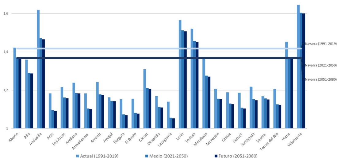
Figura 27 Evolución del riesgo frente a inundaciones
