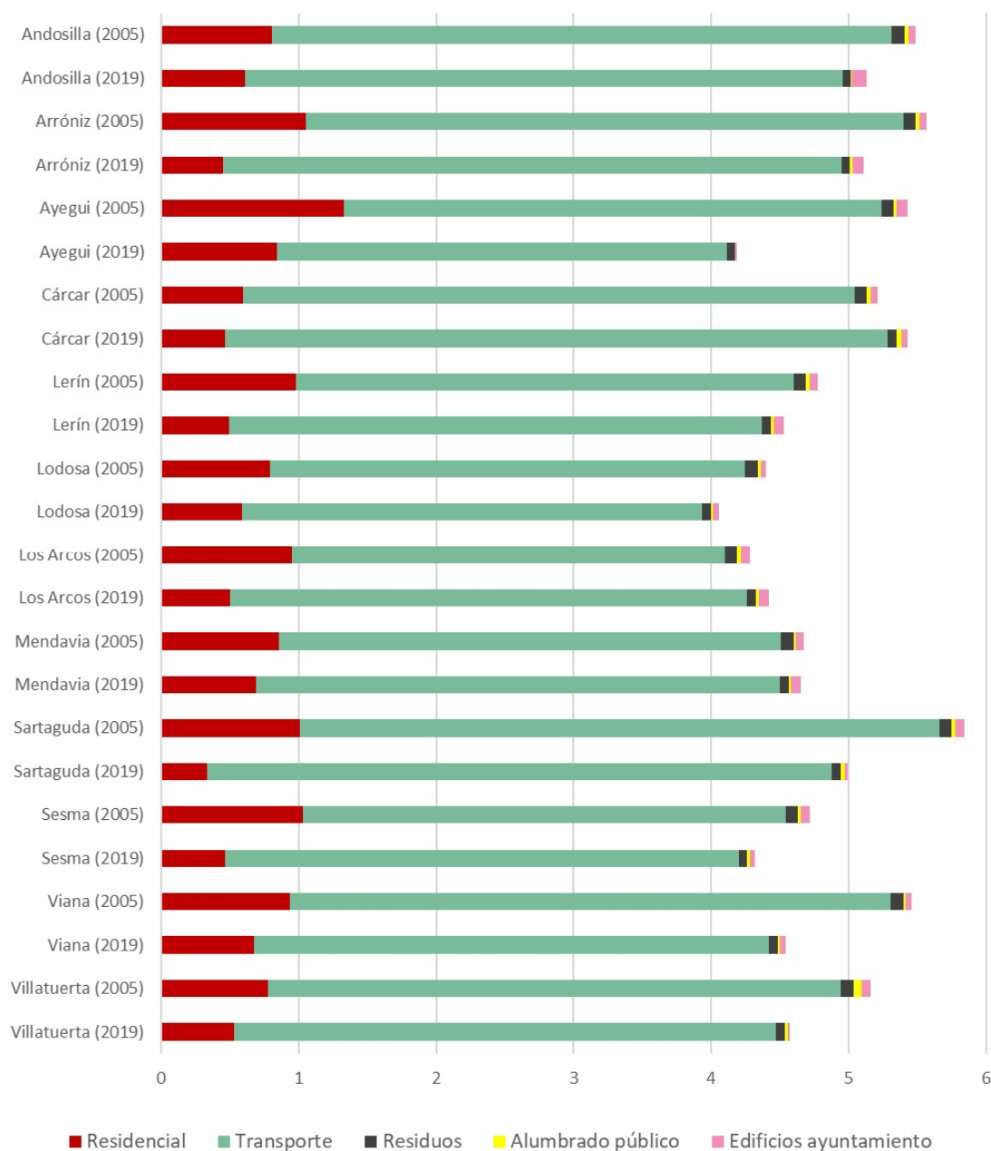
Figura 18 Evolución de las emisiones por habitante (tCO 2 /hab.), por municipio de >1.000 habitantes
