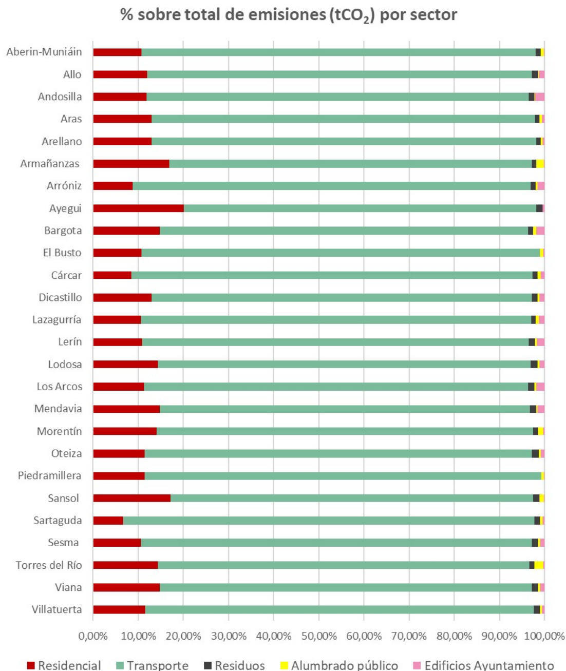
Figura 19 Distribución de emisiones (tCO 2 ) por sector sobre total del municipio, 2019
