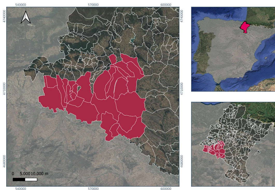
Figura 1 Localización de la agrupación, elaboración propia
