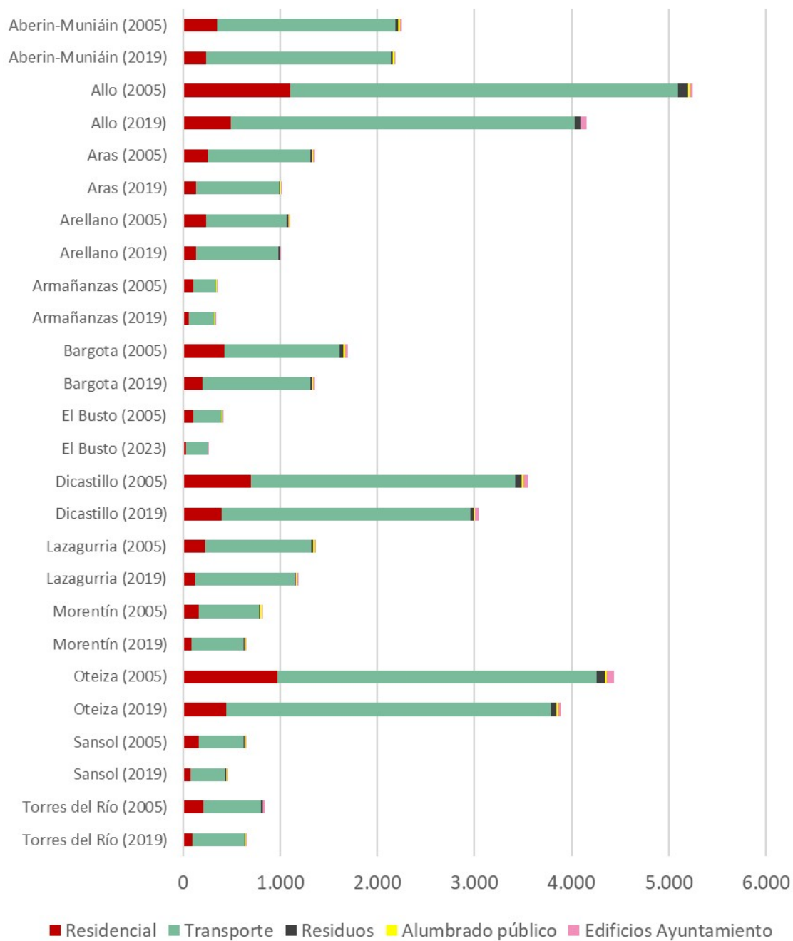
Figura 15 Evolución de las emisiones (tCO 2 ) por municipio y sector, para municipios <1.000 habitantes
