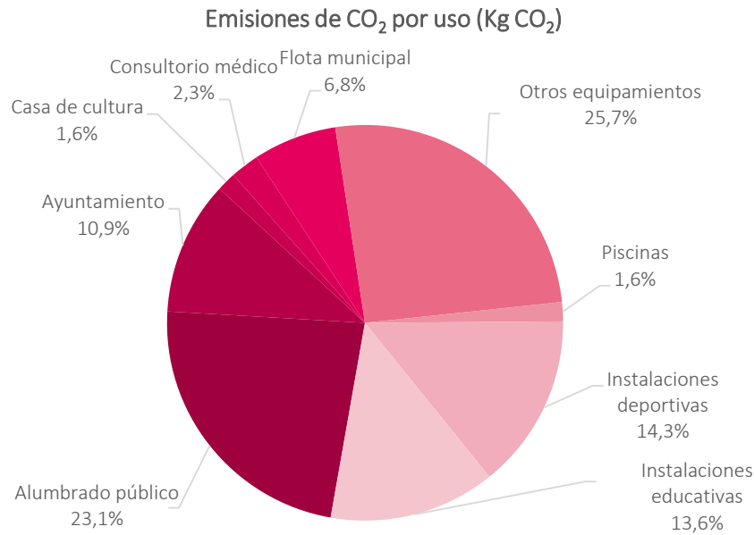
Figura 22 Emisiones municipales (kgCO 2 ) de la agrupación, % por uso
