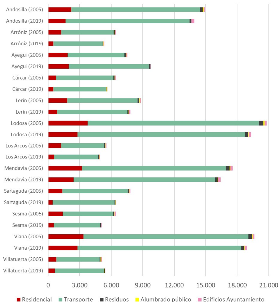
Figura 16 Evolución de las emisiones (tCO 2 ) por municipio y sector, para municipios >1.000 habitantes
