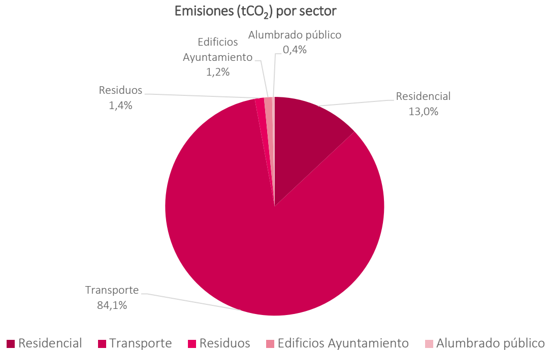
Figura 20 Emisiones (tCO 2 ) de la agrupación, por sector
