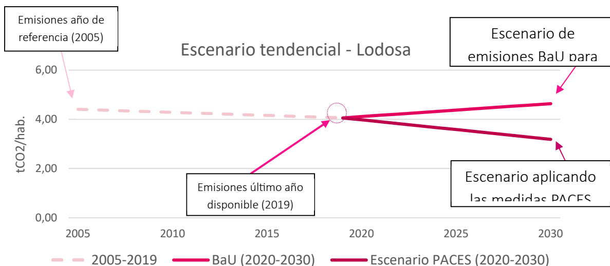
Figura 24 Ejemplo de gráfico de escenarios tendenciales 2030 del Anexo VI
