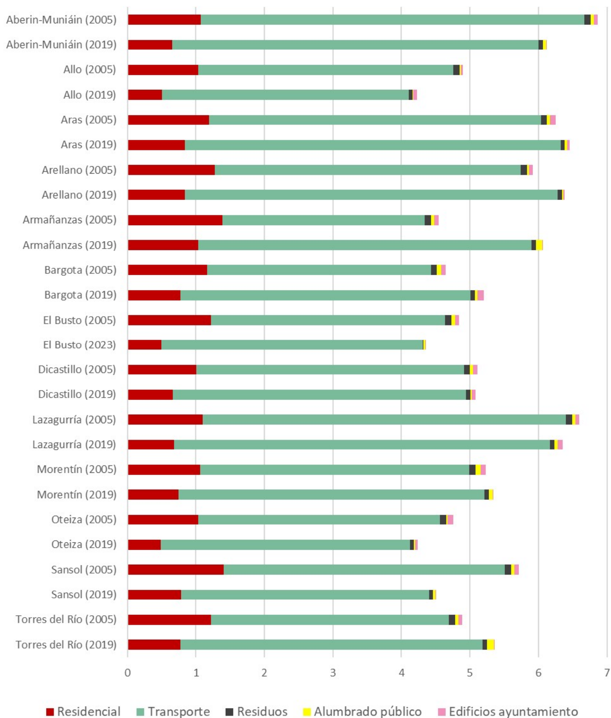
Figura 17 Evolución de las emisiones por habitante (tCO 2 /hab.), por municipio de <1.000 habitantes
