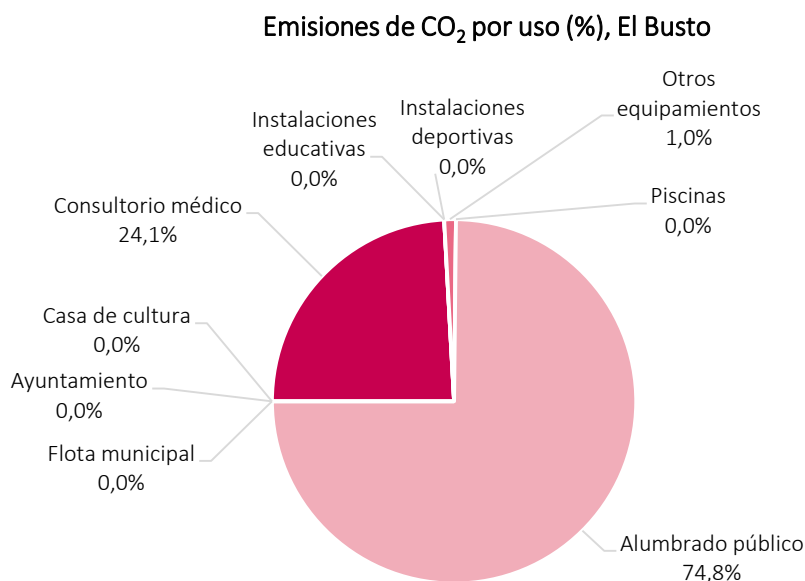
Figura 23 Emisiones municipales (kgCO 2 ) de El Busto, % por uso
