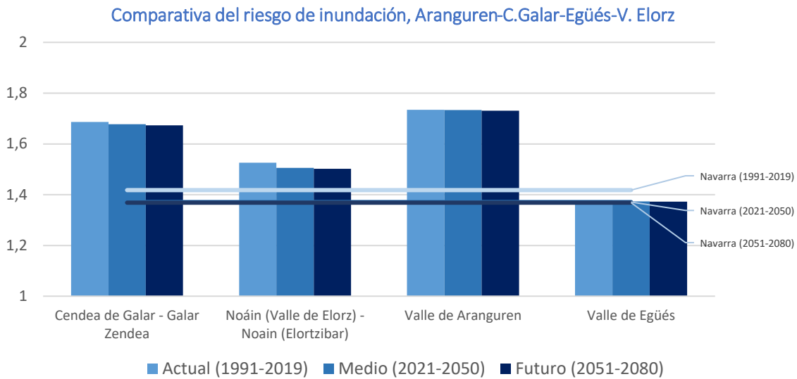
Figura 18 Evolución del riesgo frente a inundaciones
