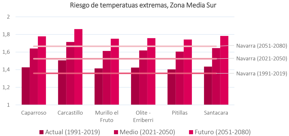
Figura 15 Evolución del riesgo frente a temperaturas extremas
