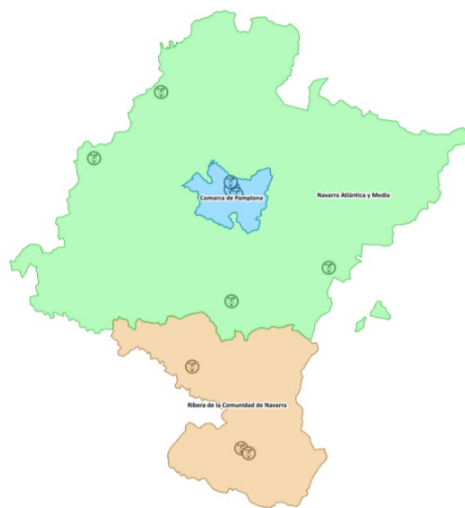
Zonificación PM10, PM2,5 y NO2
